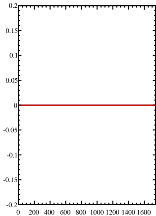
fEpsilonHist
