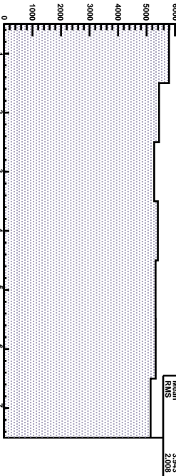
HKS AC2+ raw ADC hitpat
