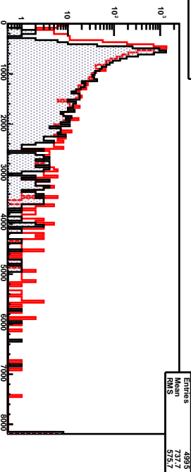
HWCI-D6 RAW ADC-
