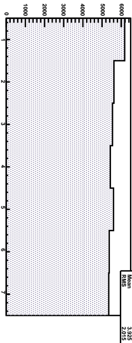
HKS AC3+ raw TDC hitpat
