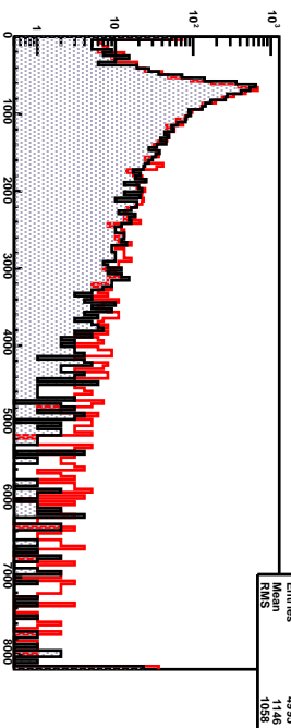
HWCI-D1 RAW ADC-
