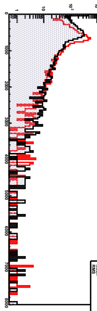
HACH-3 RAW ADC-2
