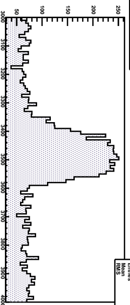
EDCZ raw tDC layer 04 xp
