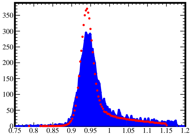
W (GeV)
