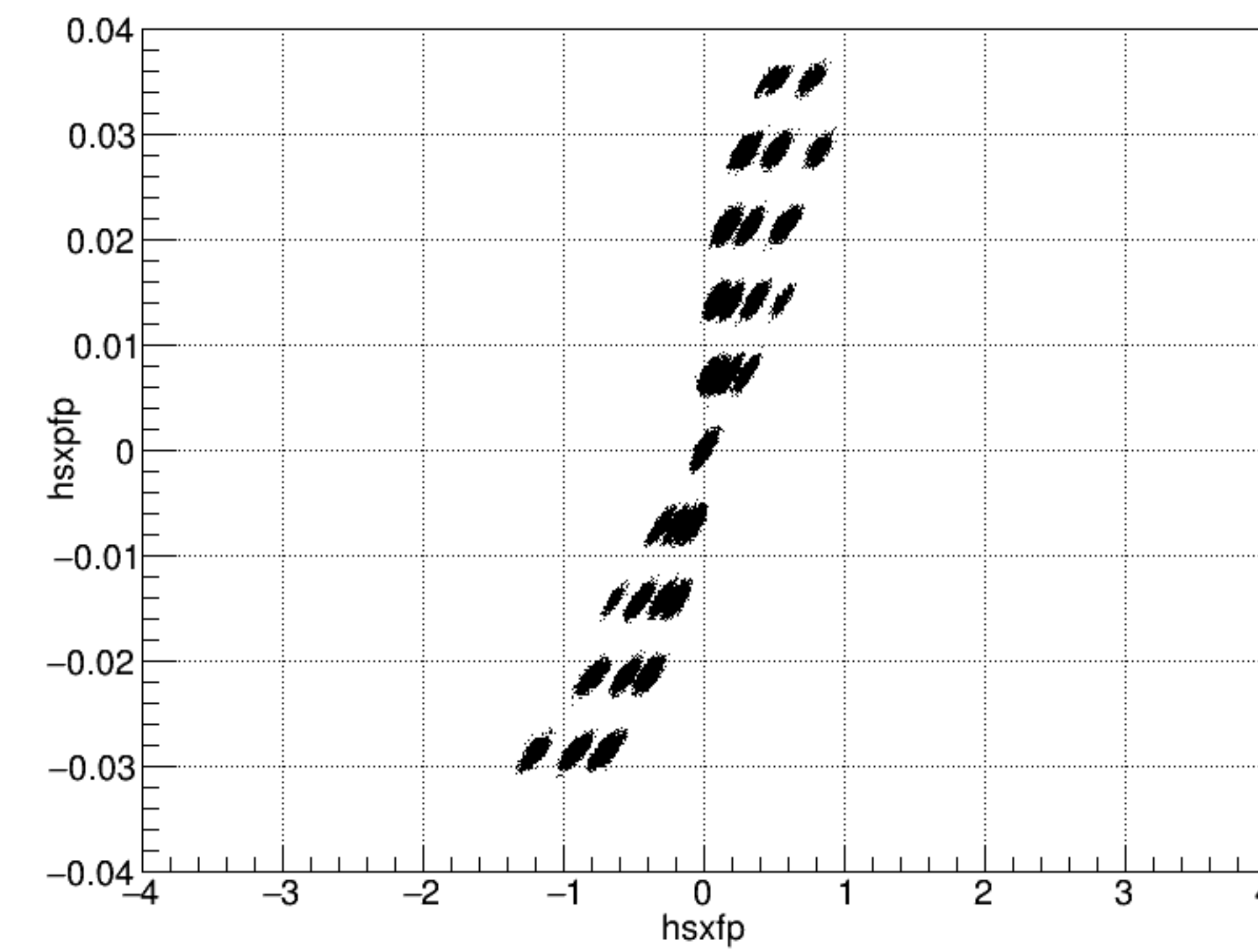
hsxpfp vs hsxfp Q1_1.00_Q2_1.00_Q3_1.00_
