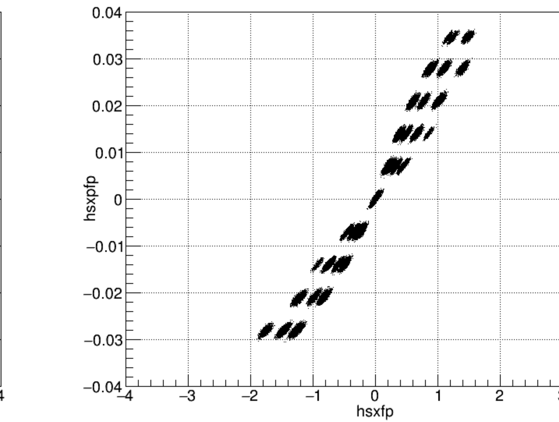
hsxpfp vs hsxfp Q1_1.00_Q2_1.02_Q3_1.00_
