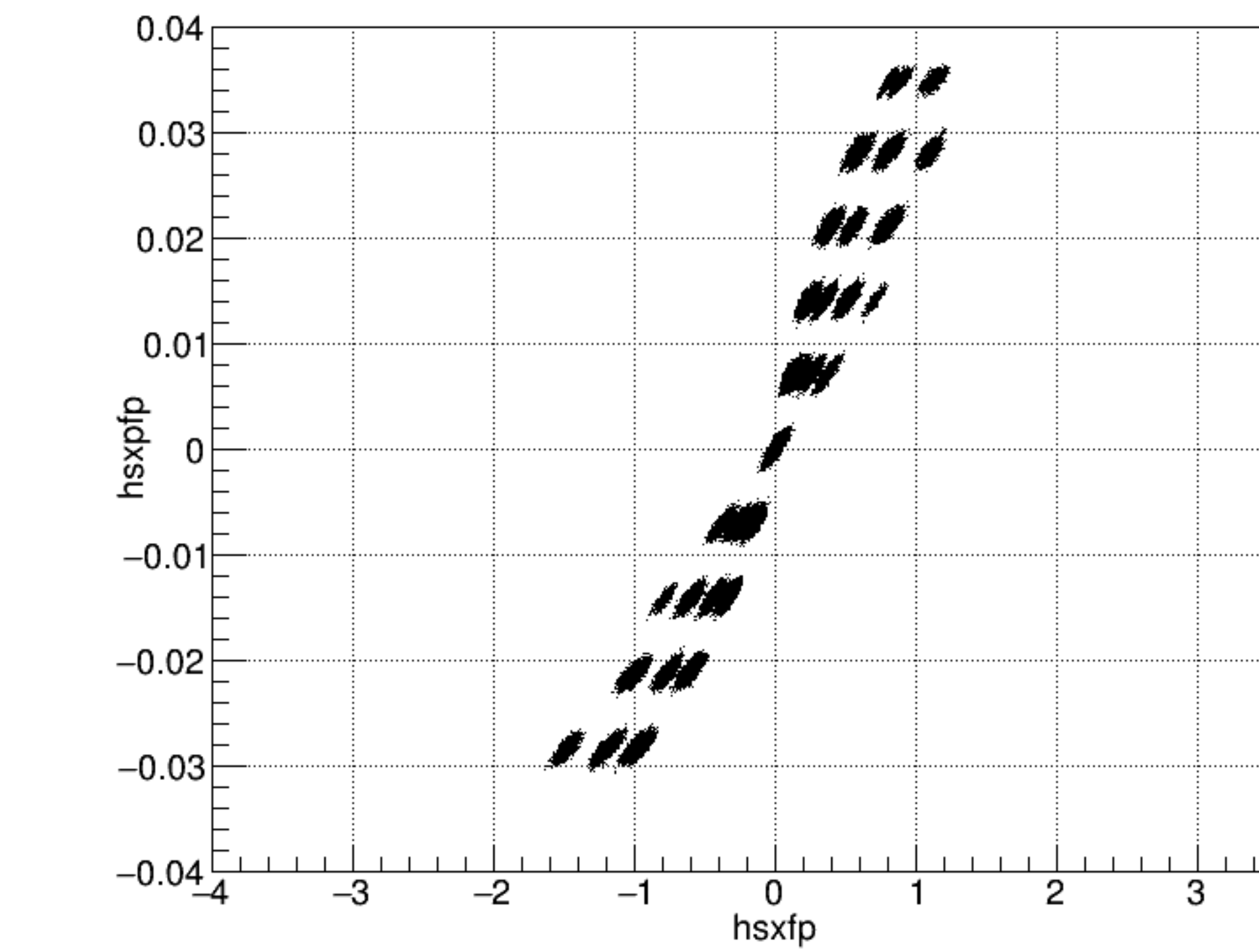
hsxpfp vs hsxfp Q1_1.00_Q2_1.01_Q3_1.00_
