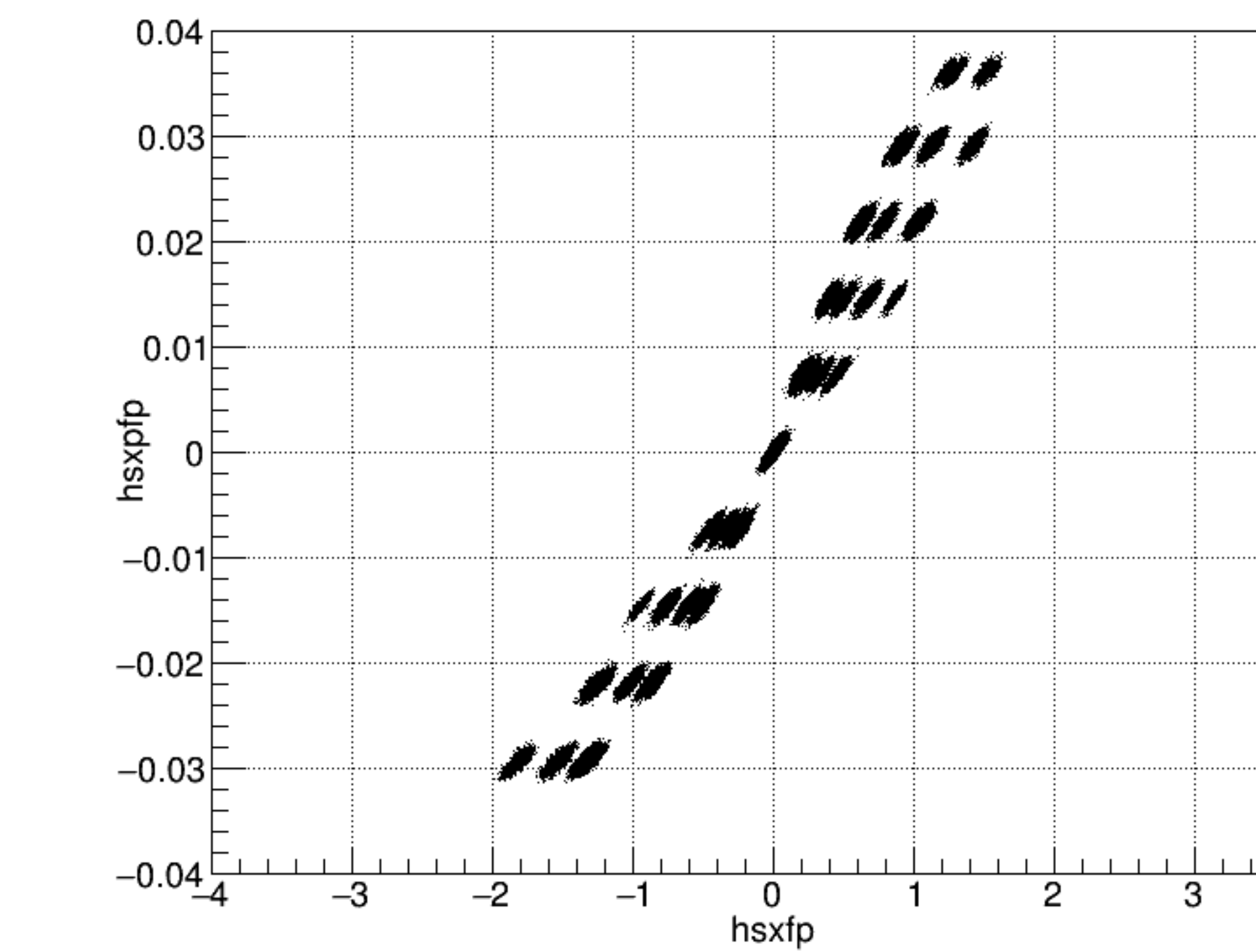
hsxpfp vs hsxfp Q1_1.00_Q2_1.00_Q3_1.01_
