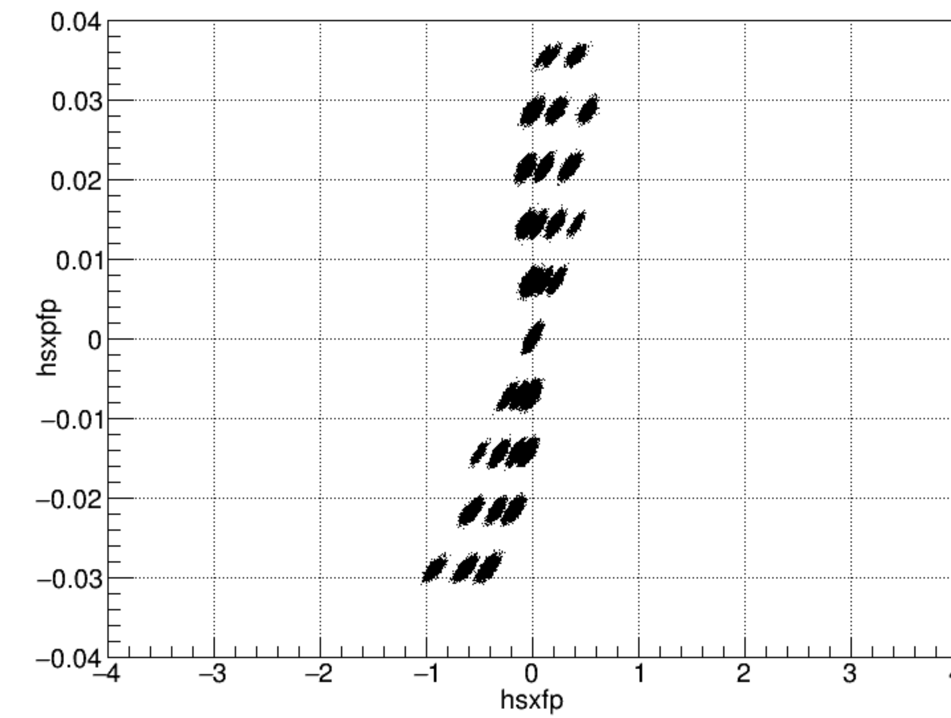
hsxpfp vs hsxfp Q1_1.00_Q2_0.99_Q3_1.00_
