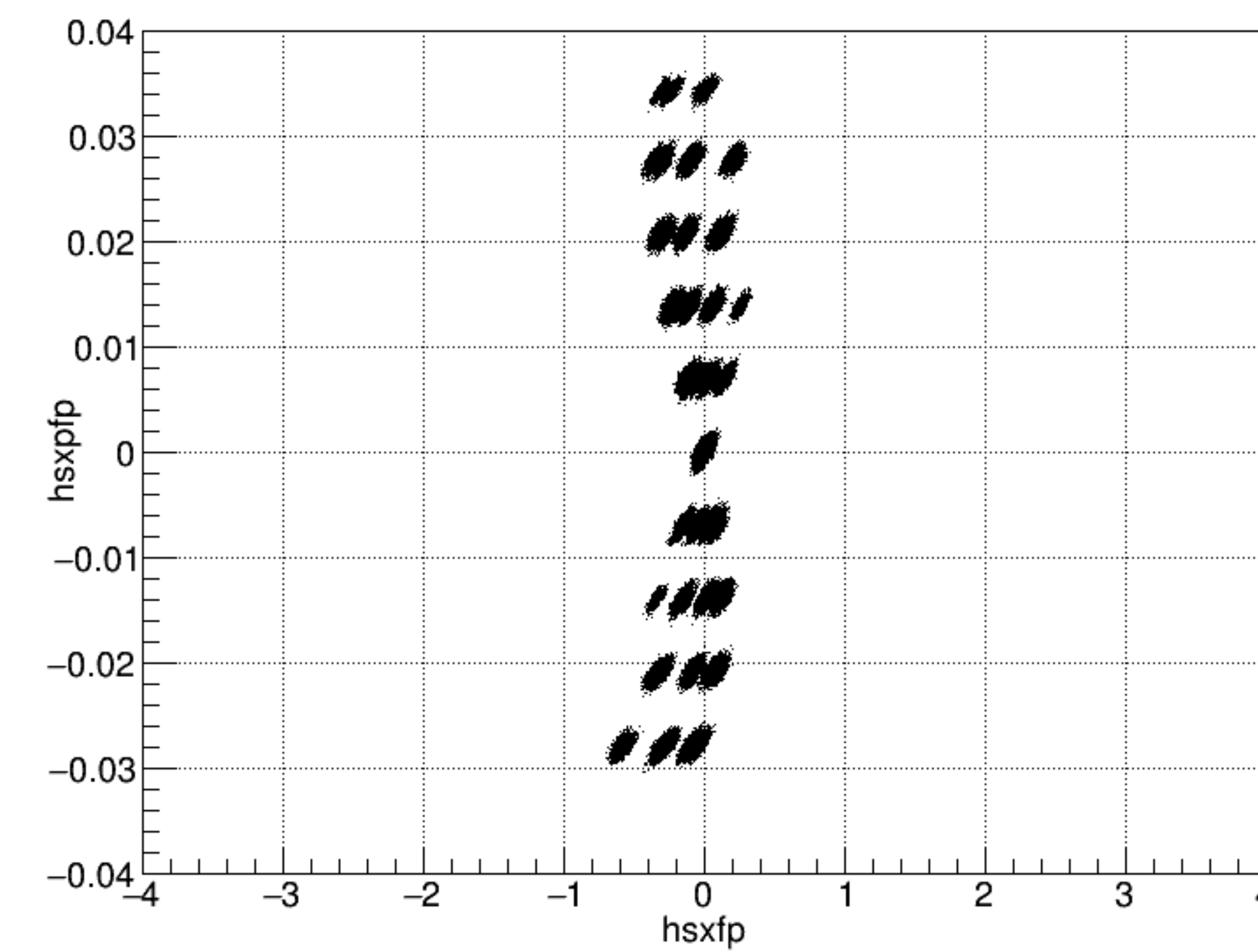
hsxpfp vs hsxfp Q1_1.00_Q2_1.00_Q3_0.99_
