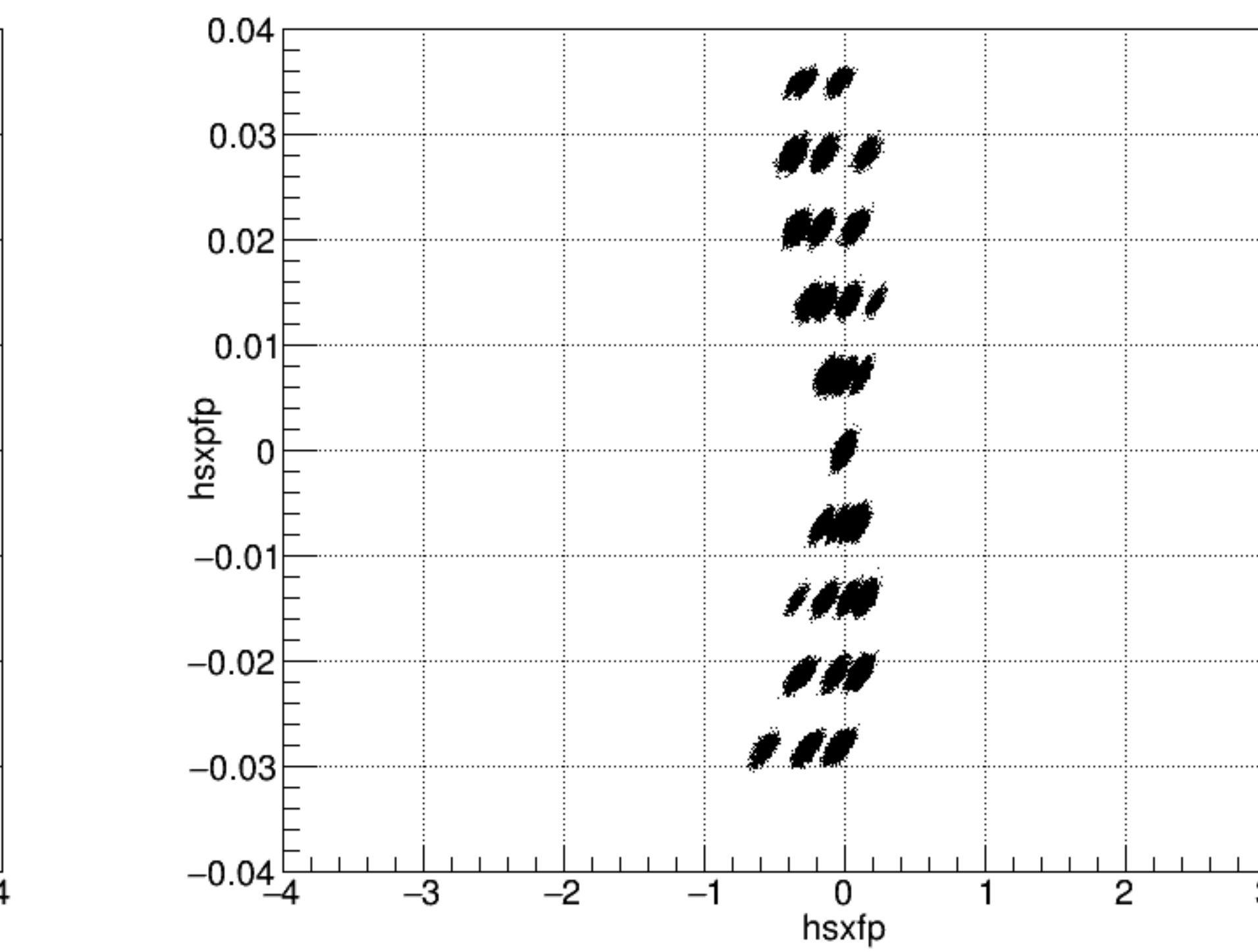
hsxpfp vs hsxfp Q1_1.00_Q2_1.00_Q3_1.02_
