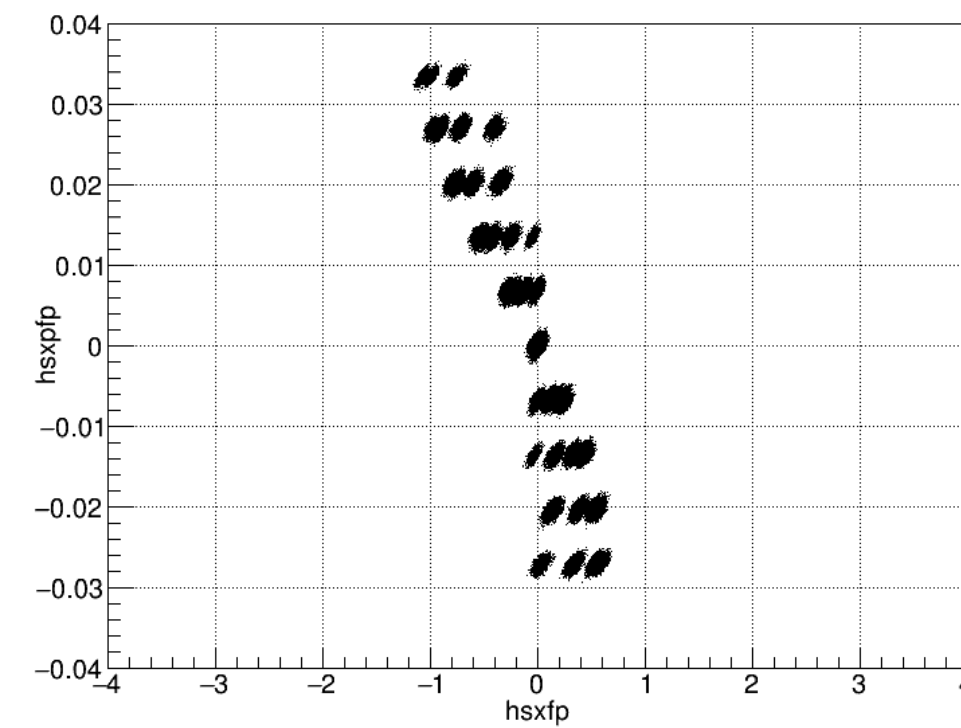
hsxpfp vs hsxfp Q1_1.00_Q2_1.00_Q3_0.98_
