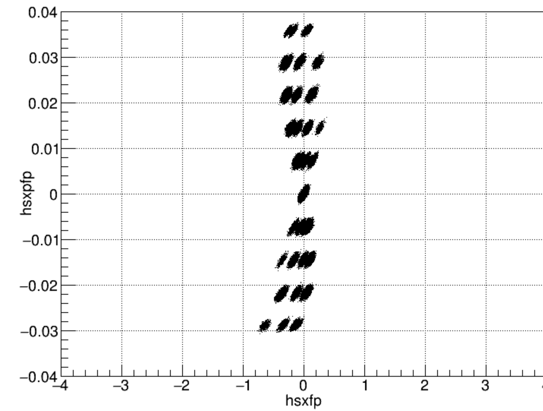
hsxpfp vs hsxfp Q1_1.00_Q2_0.98_Q3_1.00_
