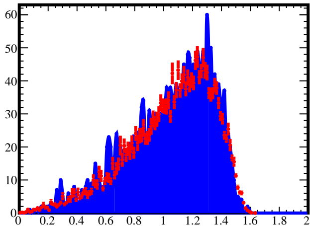
W (GeV)
