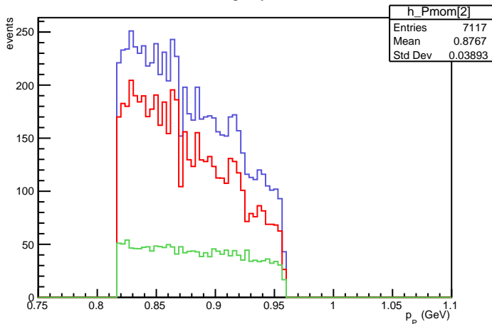
HMS mom.
