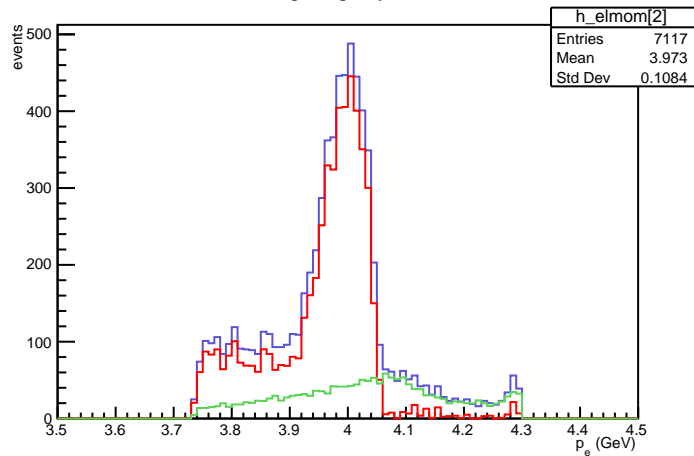
SHMS mom.
