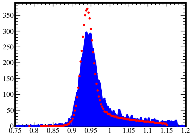
W (GeV)
