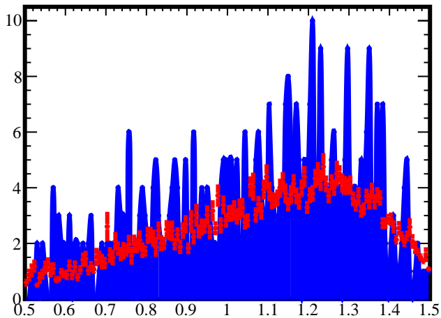
W (GeV)
